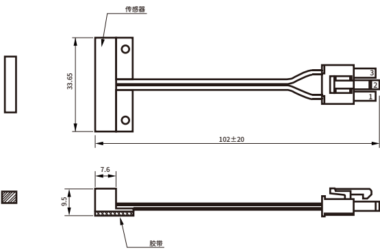
尺寸 (mm)
