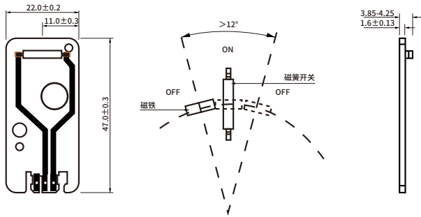
尺寸 (mm)
