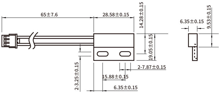
尺寸 (mm)
