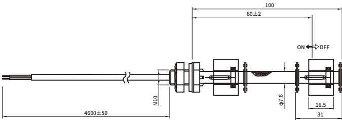
尺寸 (mm)
